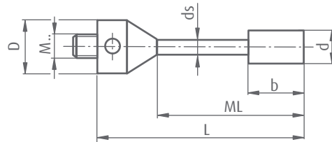
Zylindertaster
